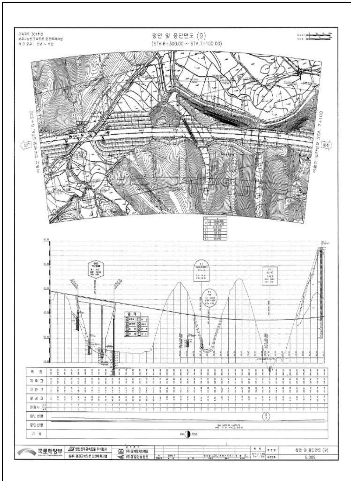
【그림 51.1.4】 평면도
